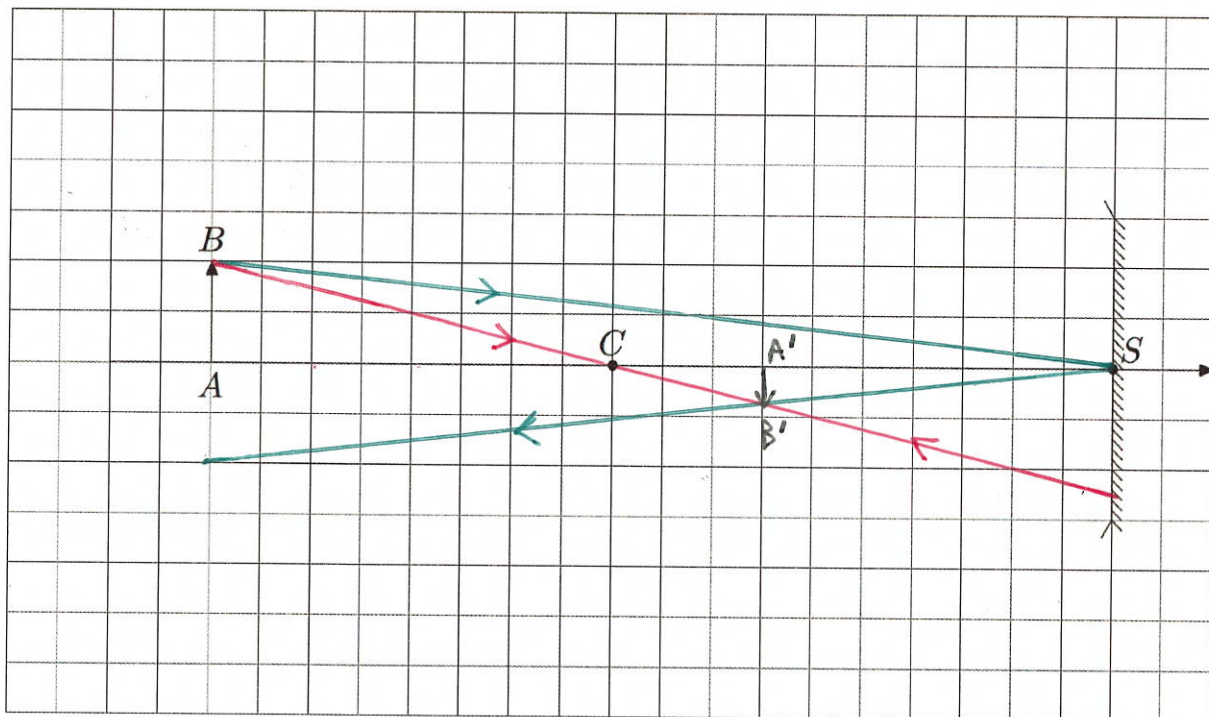
FIG. 3 – Miroir sphérique
