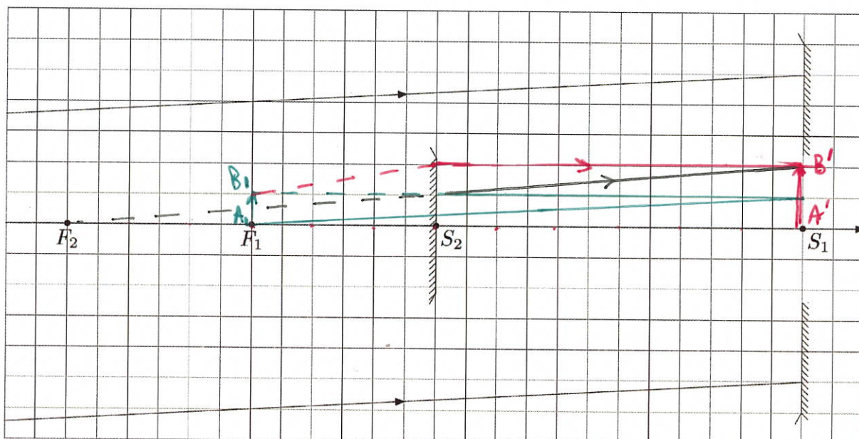
FIG. 4 – Télescope de Cassegrain
